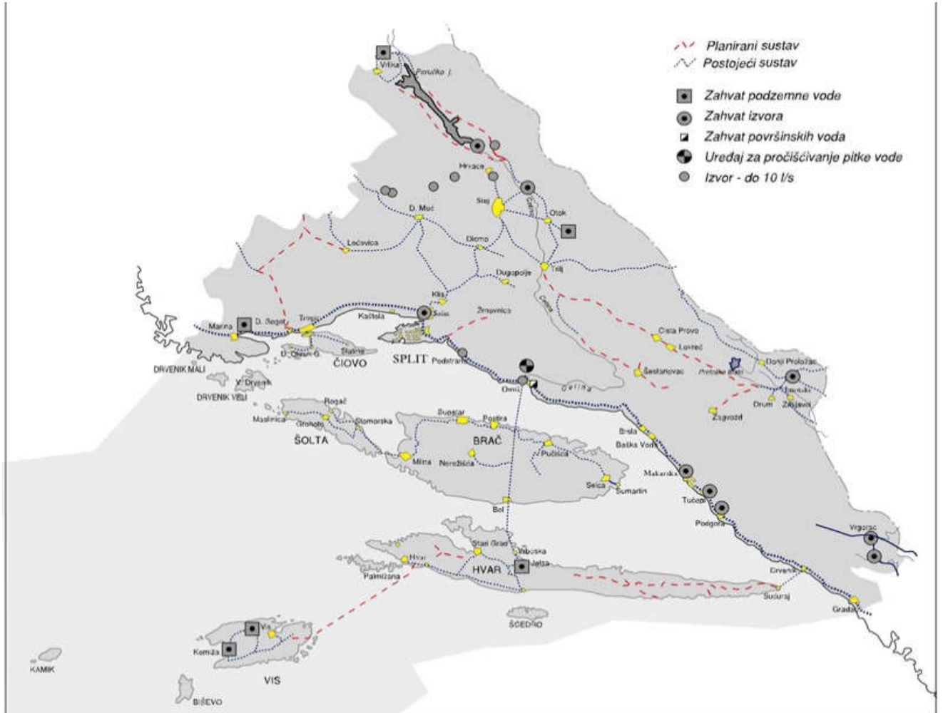
Slika 1. Vodoopskrbni sustav Splitsko-dalmatinske županije
